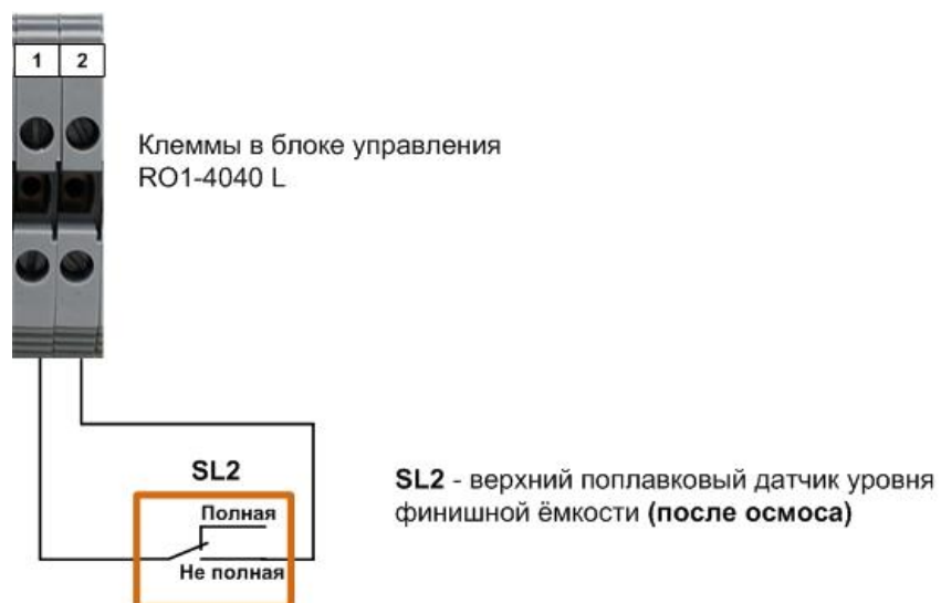
Рис. 5. Электрическая схема подключения датчика уровня к установке.
