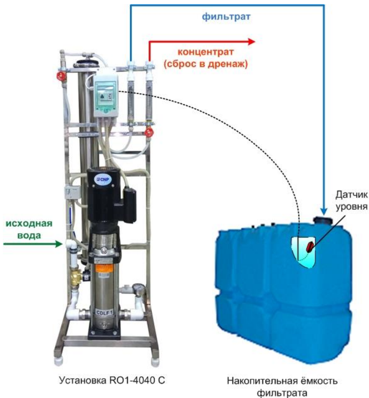
Рис. 3. Подключение трубопроводов к установке.
