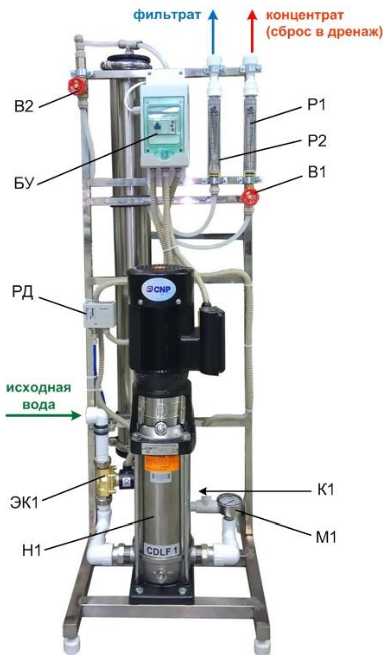
Рис.1 Общий вид установки.
